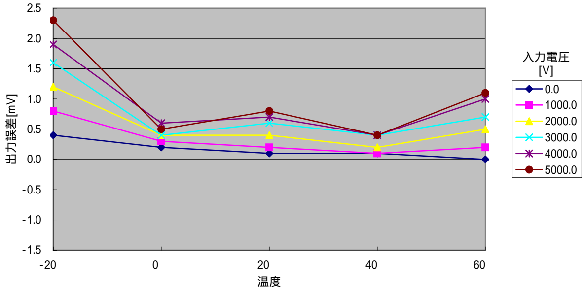
AZ05H 基板No18 温度特性
