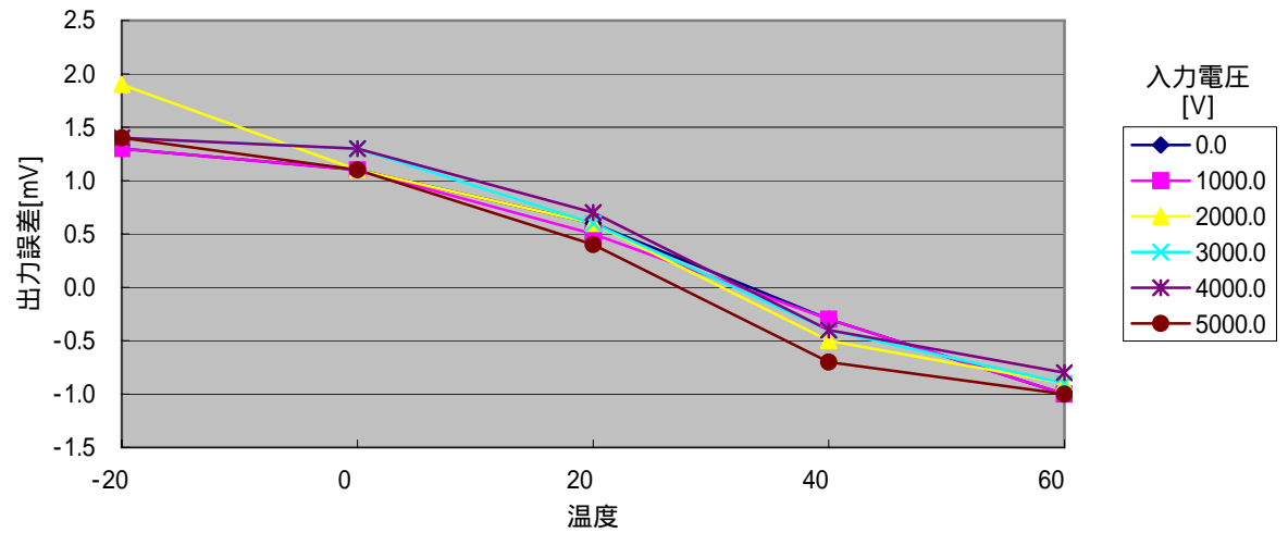
AZ05H 基板No20 温度特性
