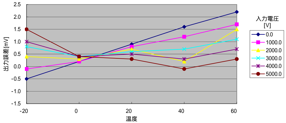
AZ05H 基板No19 温度特性
